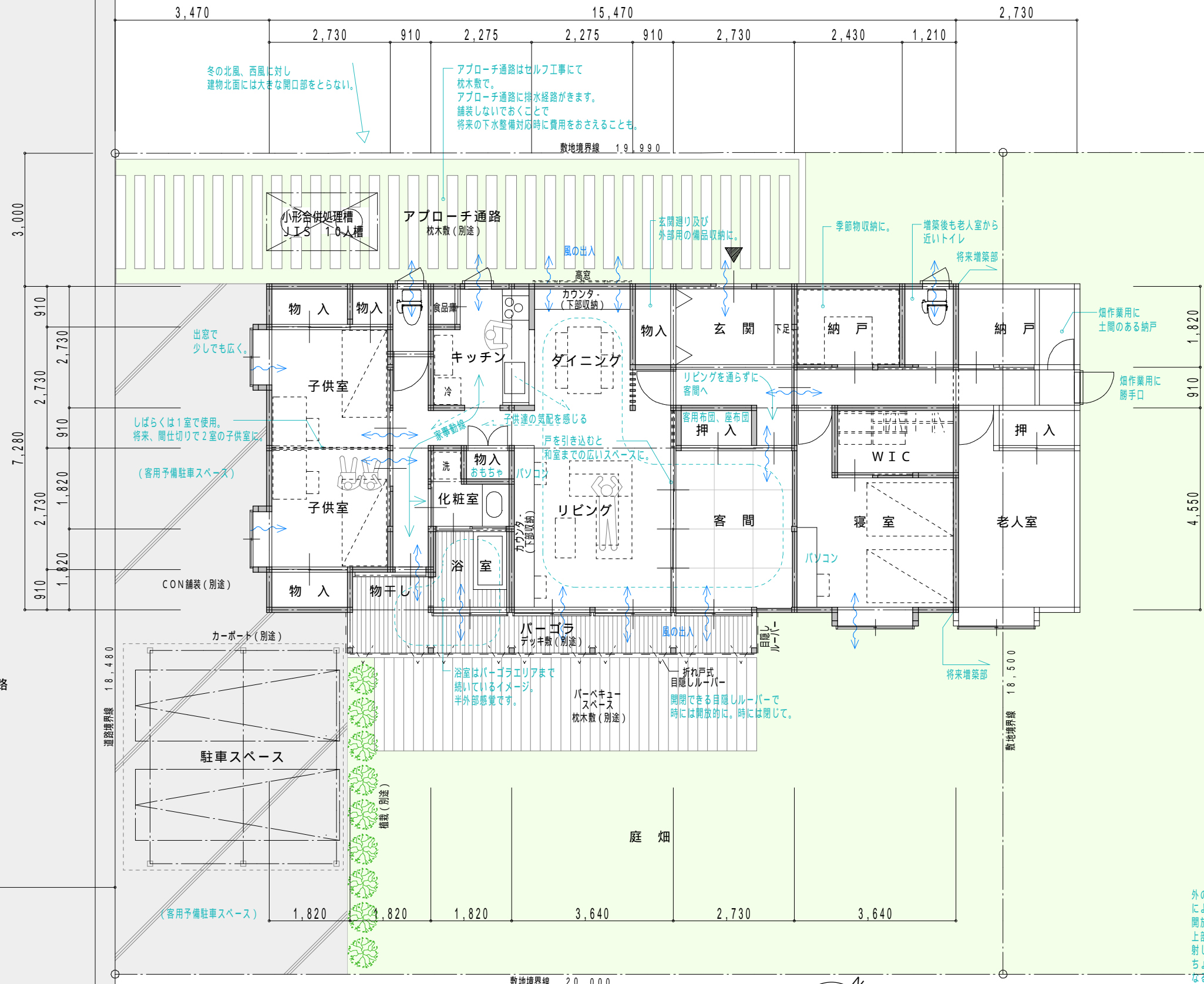
敷地境界線 20,000 配置図・平面図 1:100
